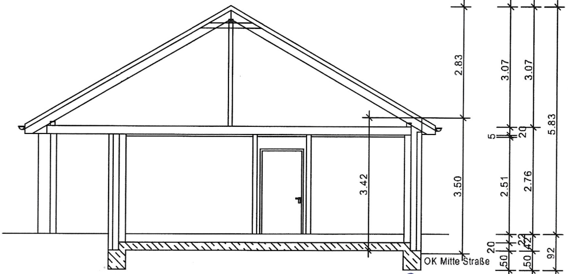
Schnitt A-A
